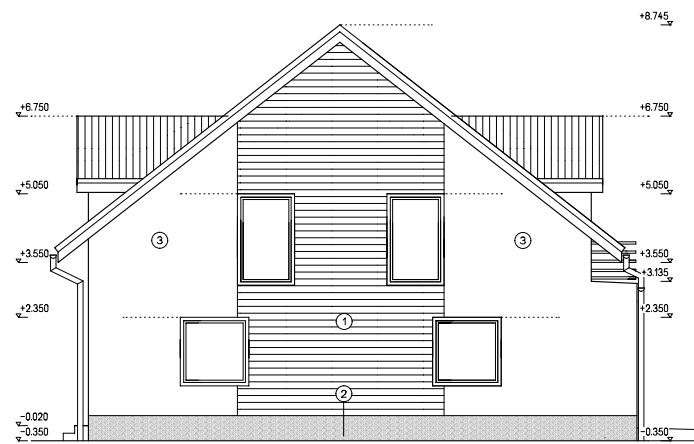
POHLED BOČNÍ
