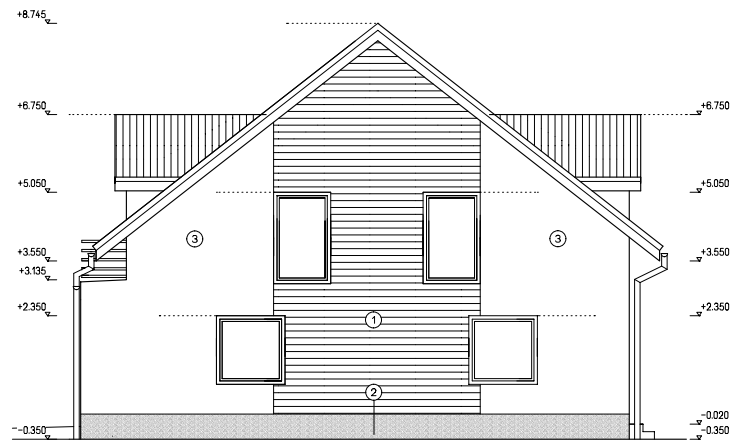
POHLED BOČNÍ
